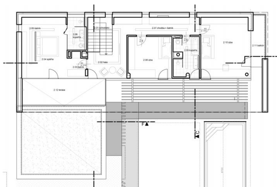
2. nadzemné podlažie
